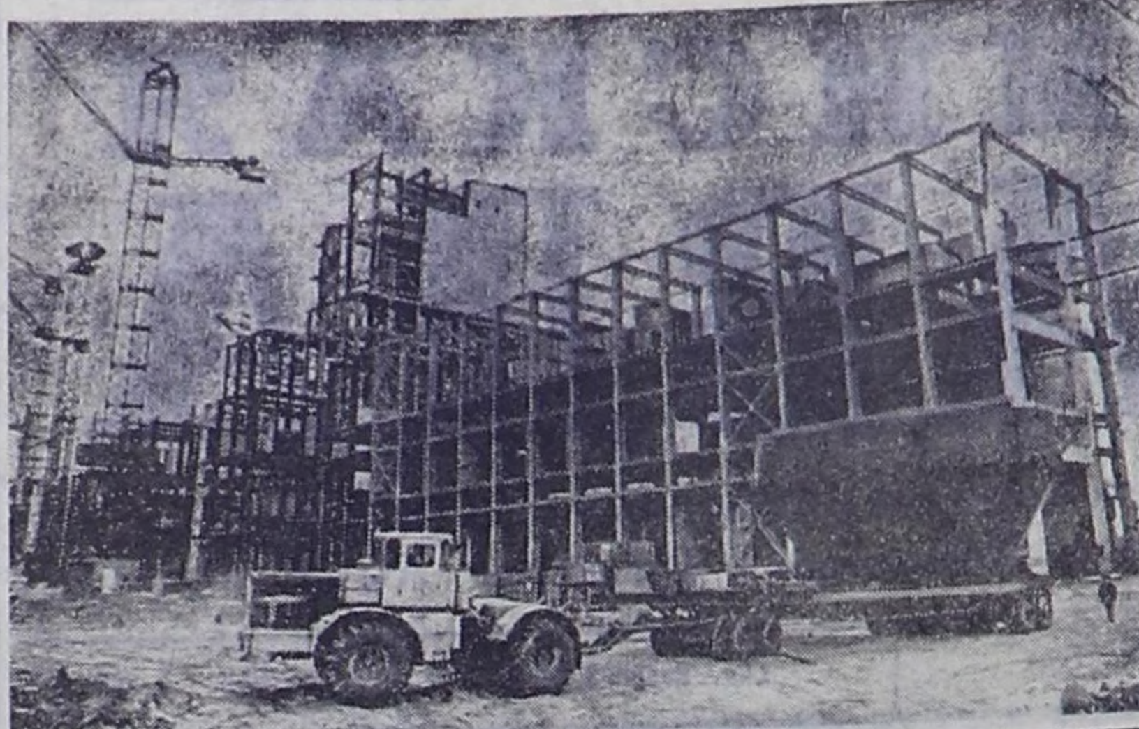
Иркутская область. Впечатляюще выглядит сегодня строительная площадка Усть-Илимского лесопромышленного комплекса. На десятках гектаров одновременно возводятся более ста различных объектов, ввод которых обеспечит современное получение первой целлюлозы уже в будущем году.
