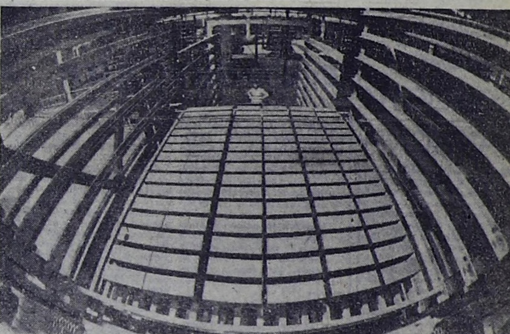
В Ярославле вступил в строй завод керамических стеновых материалов. Все процессы — от приготовления сырья до выхода готовой продукции — автоматизированы. На одной из автоматических линий производится прочные высокопустотные керамические блоки (пустоты могут занимать до семидесяти процентов объема). Новые блоки используются в строительстве жилых домов и производственных зданий областей Нечерноземья. Производство нового завода-автомата в три раза выше, чем на кирпичных заводах. На снимке: накопитель сырого изделия на автоматической линии по производству керамических стеновых материалов. Фото С. Метелицы. (Фотохроника ТАСС).
