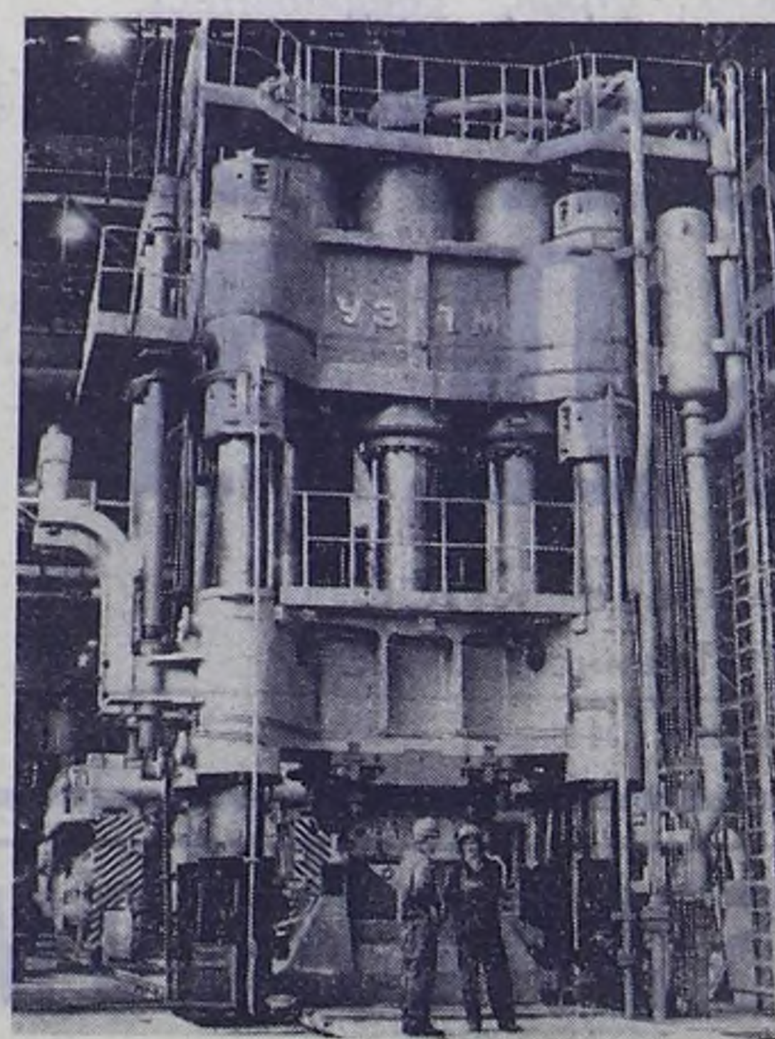
Свердловск. На «Уралмаше» пущен гидравлический пресс усилием четыре тысячи тонн-сил. Гигант четырех-производительного агрегата, стоявшего здесь прежде. Новая техника позволит увеличить производство поковок почти на пятнадцать тысяч тонн в год.
