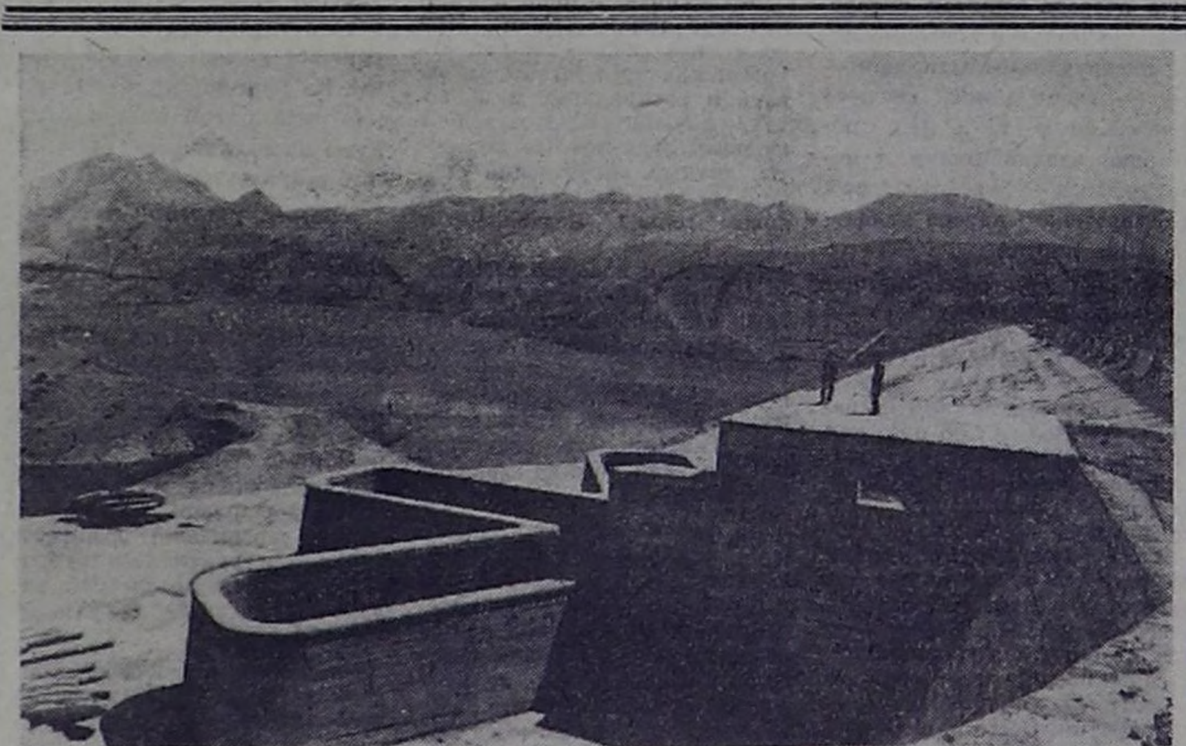
Армянская ССР. Завершается строительство Азатского водохранилища — одного из крупнейших в Армении. В искусственном озере, зеркало которого составит почти три квадратных километра, будет собрано 70 миллионов кубических метров воды.
