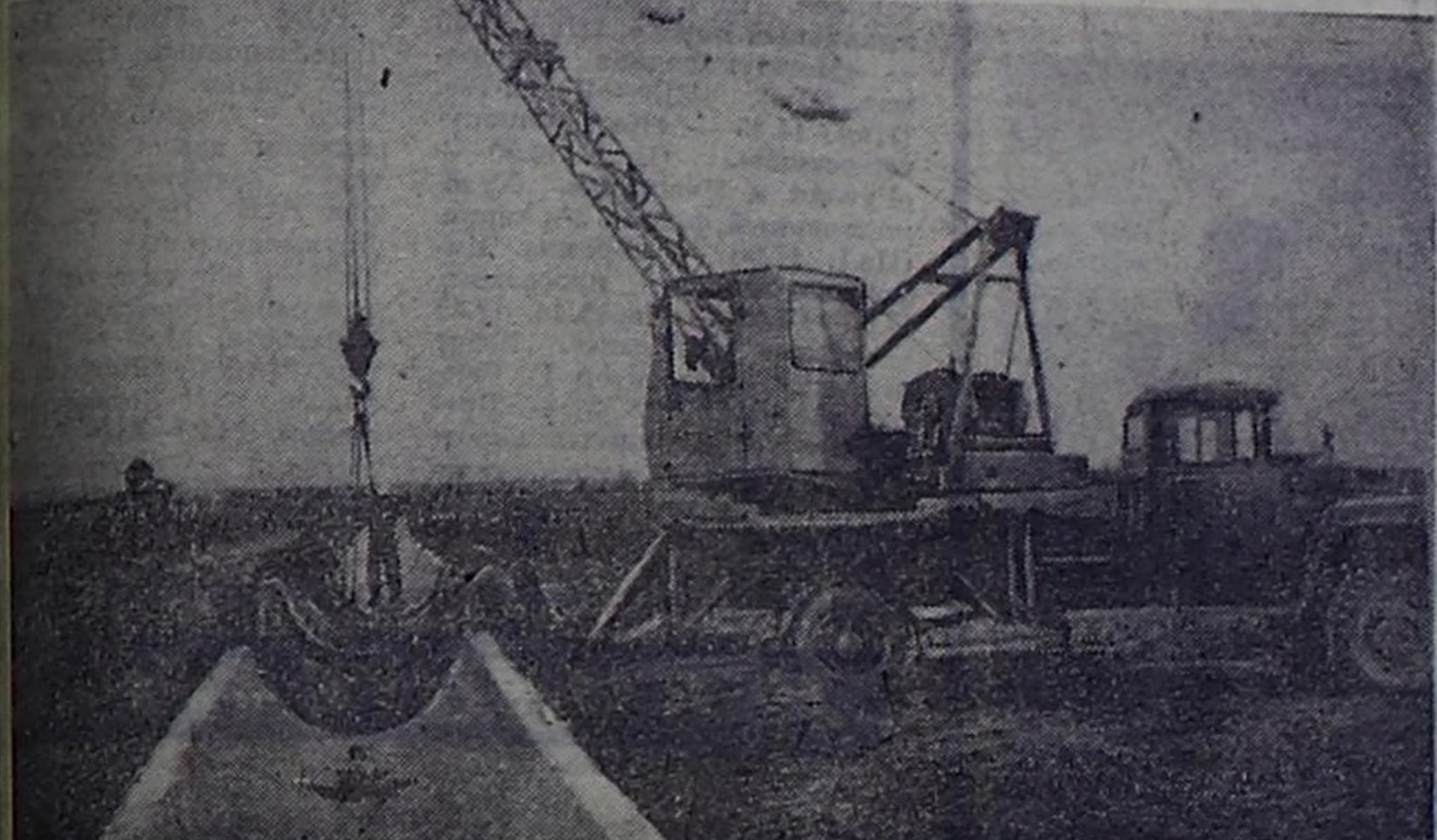
Первые в Туве при реконструкции Элегейтинской оросительной системы строители ПМК-2 треста «Тувинводстрой» монтируют железобетонные лотки. Лучшая бригада монтажников ПМК-62, руководит которой Г. А. Елизаров, уже выполнила лотками два канала общей протяженностью 1 километра (на снимке слева). Выгода примененного
