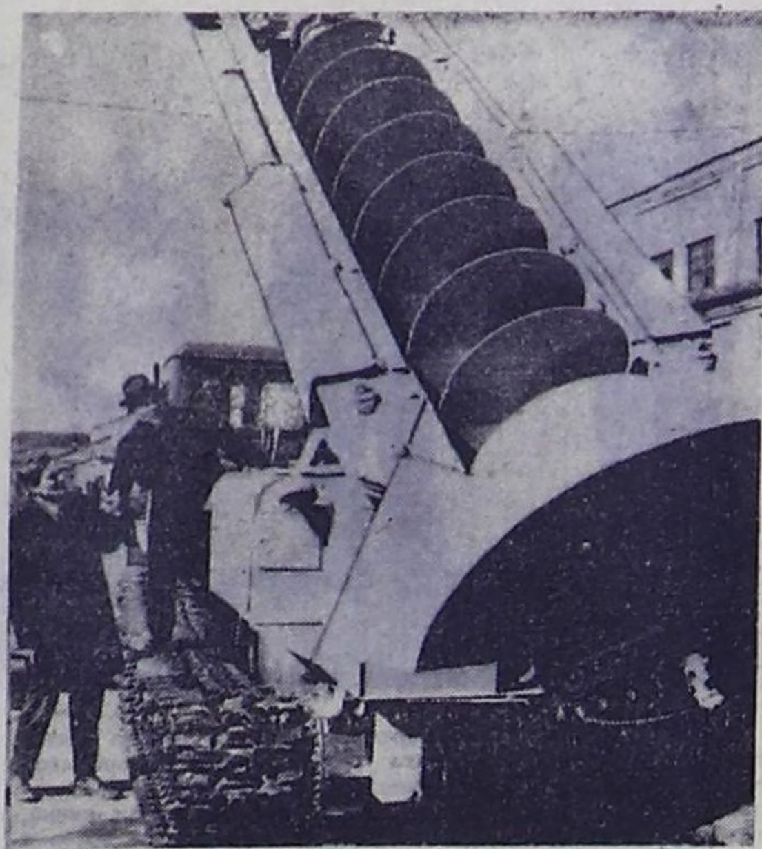
Иваново. Механический завод «Главэнергостроймеханизация» приступил к серийному выпуску машин МРК-750Т, предназначенных для рытья котлованов под опоры линий высоковольтных электротрансформаторов. На котлован глубиной до 3,5 метра и диаметром 750 миллиметров с помощью агрегата ТТ-4, что позволяет работать в местах с повышенной влажностью. На снимке: ведущий конструктор машины Ю. М. Носов (слева) и один из авторов нового бора инженер-конструктор Г. Г. Горохов осматривают машину после заводских испытаний.
