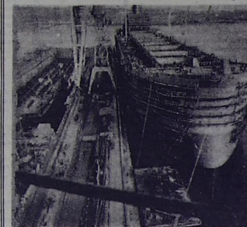
Польша. На верфи имени Парижской коммуны в Гдане сооружается гигантское сухогрузное судно водоизмещением 105 тысяч тонн (на с. и м. в.). В сентябре нынешнего года после окончательной отделки судно передадут советскому заказчику. На стальном корпусе 245-метровой длины будет ярко выделяться название корабля «Семен Буденный». Дальность плавания судна — 20 тысяч морских миль при скорости 16 узлов в час. Сердце морского гиганта — двигатель мощностью 23.300 л. с. — сконструировано и построено в Польше. Его работой будет управлять из центрального контрольного отделения один человек. Создатели корабля проявили максимум заботы об экипаже. Его каюты и все служебные помещения оборудованы установками искусственного климата. Фото ЦАФ—ТАСС.
