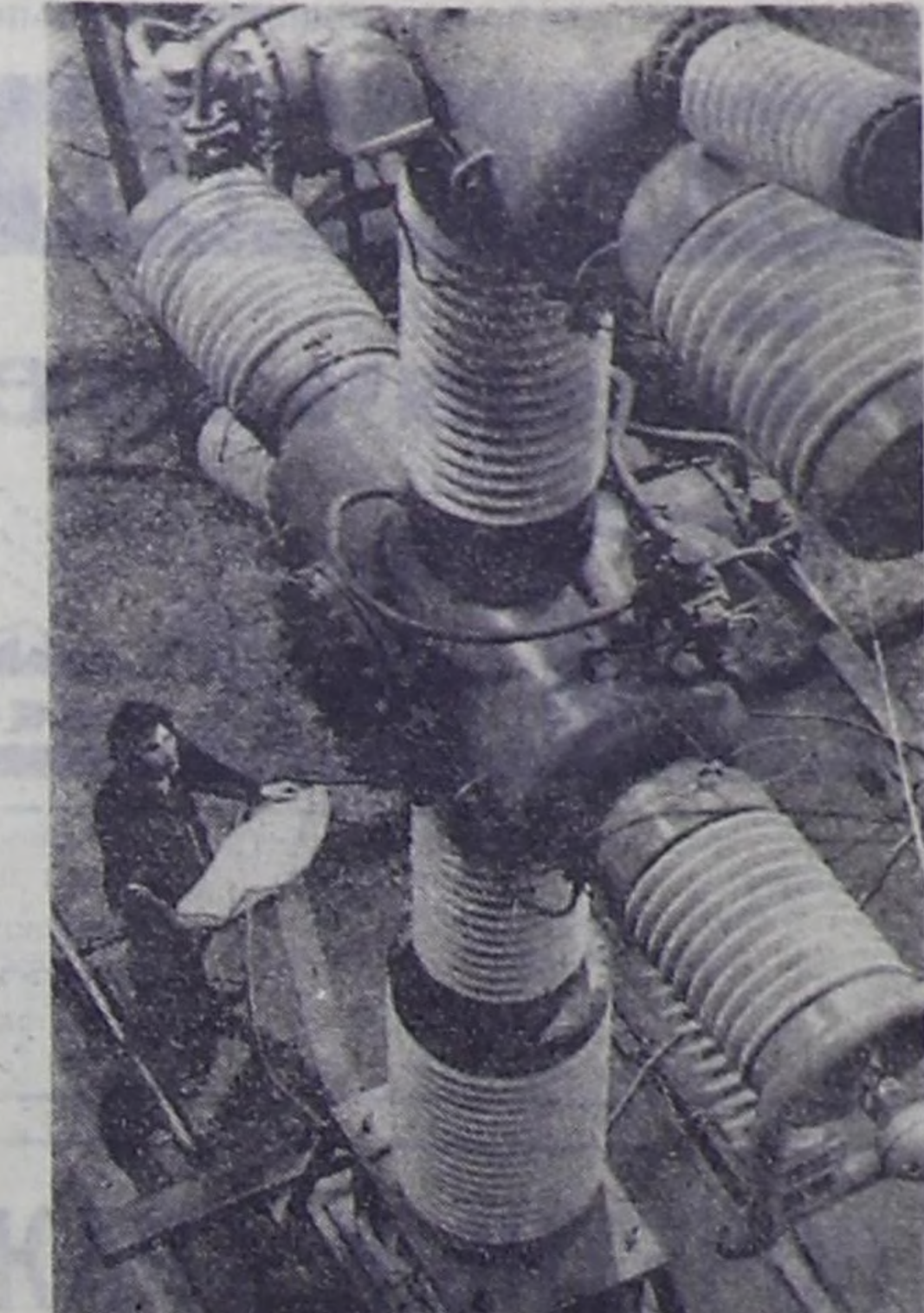
К выпуску серии холодильных выключателей для Усть-Илимской ГЭС приступил коллектив Ленинградского научно-производственного объединения «Электроаппарат». На снимке: холодильный выключатель «ВВБ-220Х1» на испытаниях в высоковольтной лаборатории «Электроаппарат».
