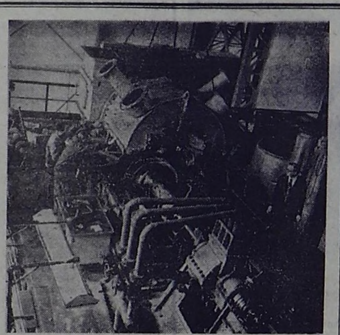
Модель турбины-гиганта
