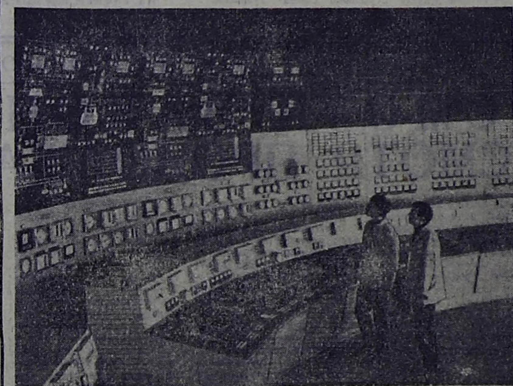
Коллектив Нововоронежской атомной электростанции на три месяца раньше срока освоил проектную мощность четвертого энергоблока. Агрегат пущен на полную мощность — 440 тысяч киловатт. На снимке: блочный пил управляет четвертым энергоблоком. (Фотохроника ТАСС).
