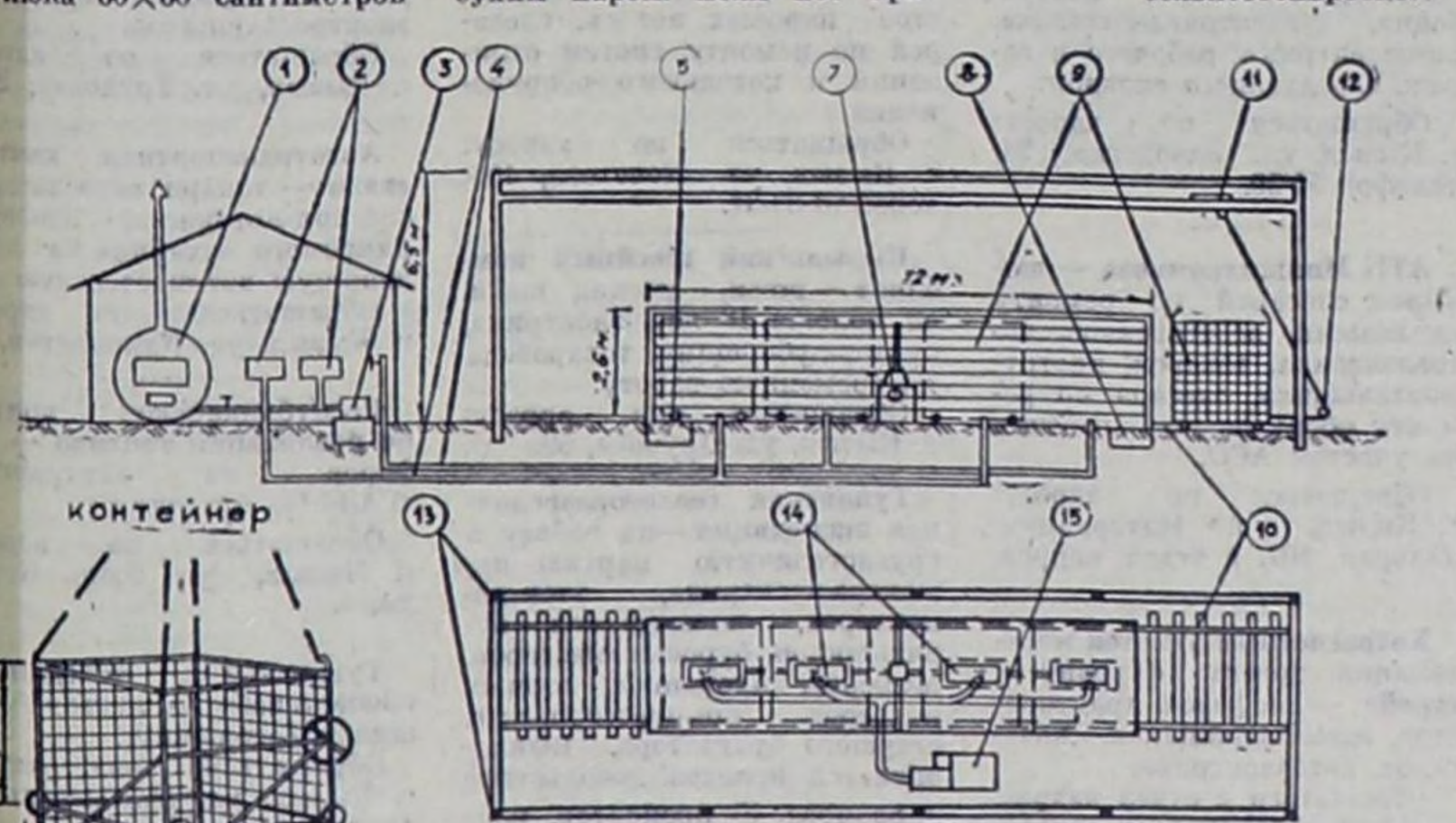
схема механизированной установки для химической и тепловой обработки соломы
