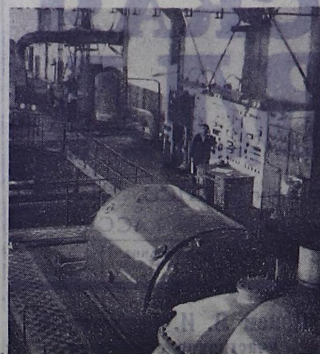
В турбинном отделении котлотурбинного цеха Кызылской электростанции.
