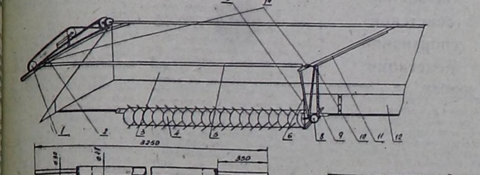
Схема жатки «ЖВН-6» с приспособлением для переворачивания валков 1. Шкив d=270 (с привода вентилятора). 2. Ремень l=3150. 3. Жатка «ЖВН-6». 4. Подборщик. 5. Вал привода подборщика. 6. Стойка l=800. 7. Кронштейн крепления подборщика. 8. Звездочка 17 зуб. (с привода подборщика). 9. Цепь, шаг 19,05. 10. Звездочка 13 зуб. (с привода трохота). 11. Кронштейн. 12. Шток. 13. Растяжка. 14. Подшипник скользящий (с вала мототила).
