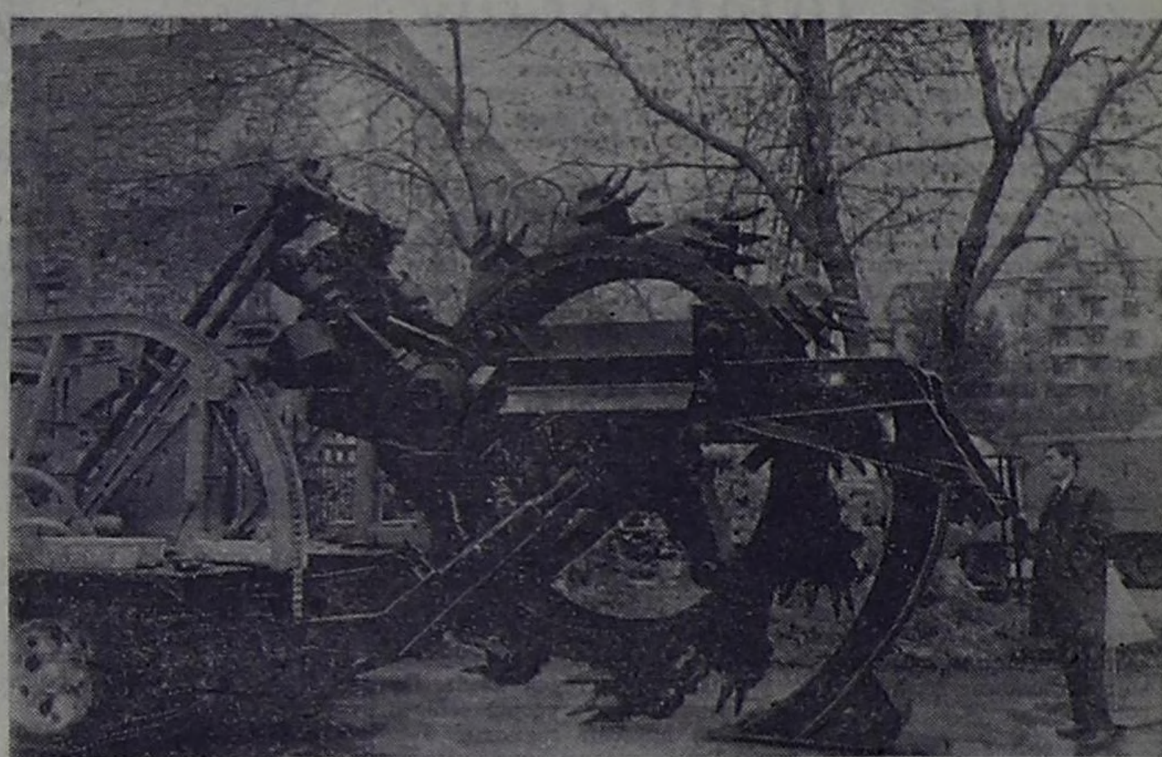
Москва. На ВДНХ СССР в разделе «Строительство» на Фрунзенской набережной открыта тематическая выставка «Машины для разработки мерзлых грунтов». На ней демонстрируются новые мощные экскаваторы, бульдозеры, фрезерные машины. На снимке: роторный экскаватор «БТМ-ТМГ», предназначенный для рытья траншей в талых и мерзлых грунтах. За час работы в мерзлых грунтах он образует траншею длиной до 200 метров и глубиной в 1,5 метра. Изготовлен на Дмитровском экскаваторном заводе Министростройа. Разработан СКБ Мосстроя Главмостроя. Фото Н. Кулепова. (Фотохроника ТАСС).
