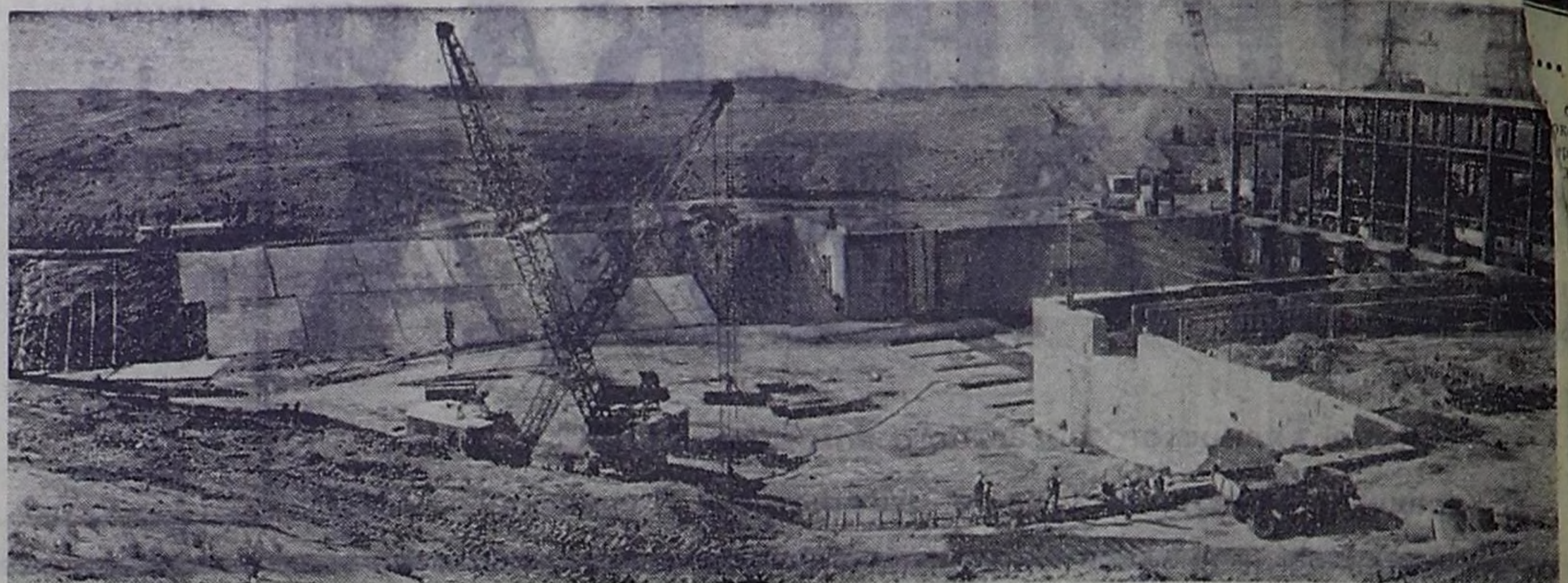
Уабекская ССР. Краем безмолвия называли некогда Каршинскую степь. Теперь она оживает деловитым рокотом моторов. Здесь сооружается магистральный машинный канал протяженностью 200 километров, на берегах которого раскинется новая хлопковая долина. Воду из Амударьи подведут на обширные плантации шести насосных станций.
