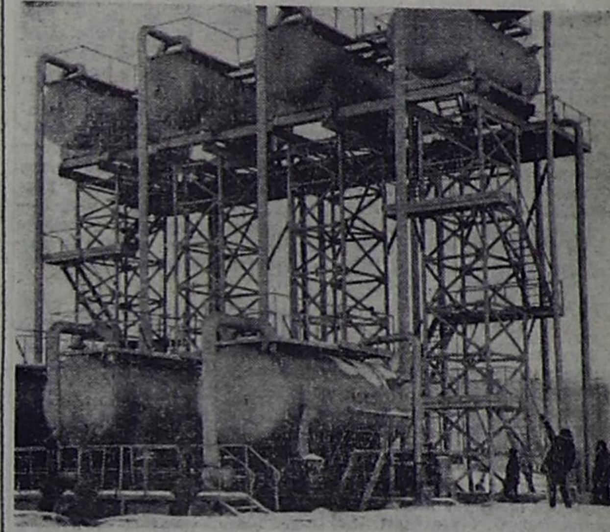
На Западно-Сургутском месторождении нефти вступила в строй мощная сепарационная установка. Ее производительность несколько тысяч тонн нефти в сутки. Установка позволила улучшить качество нефти.
