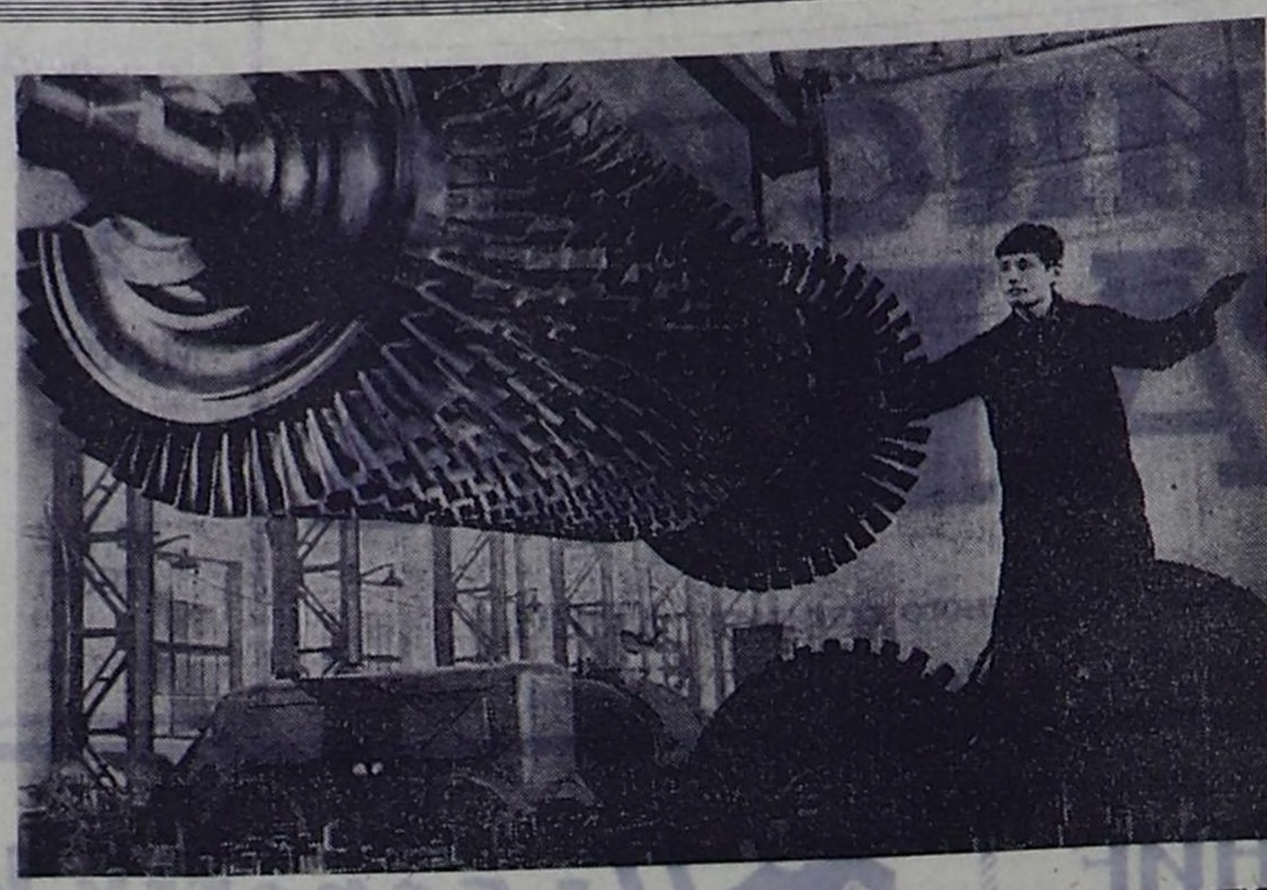
Свердловск. Уральский турбомоторный завод изготавливает газовые турбины для компрессорных станций трубопроводов. Выполняя обязательства, взятые в честь XXIV съезда КПСС, рабочие и специалисты предприятия досрочно собрали турбину, предназначенную для газопровода Пермь—Серов.
