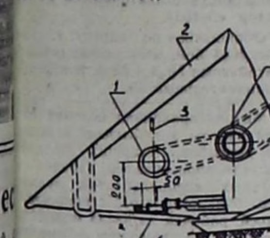
Рис. 2. 1-Звездочка 2-45 2-Корпус жатки 3-Планка мотопилы 4-Звездочка шнека жатки 5-Звездочка 2-10 ведущая 6-Пальцевый брус мотопилы
