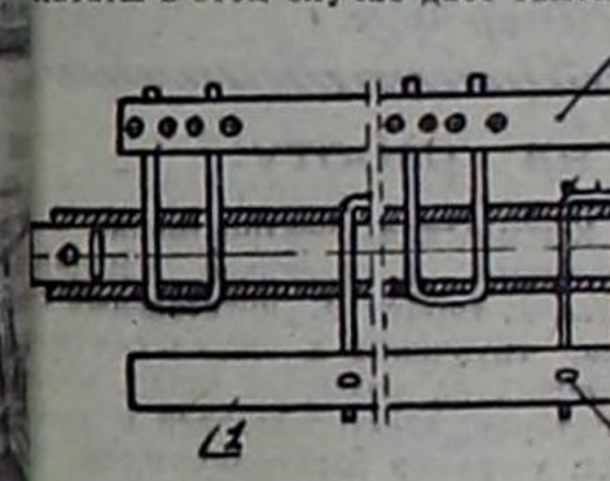
Рис. 1. Планка мотопилы
