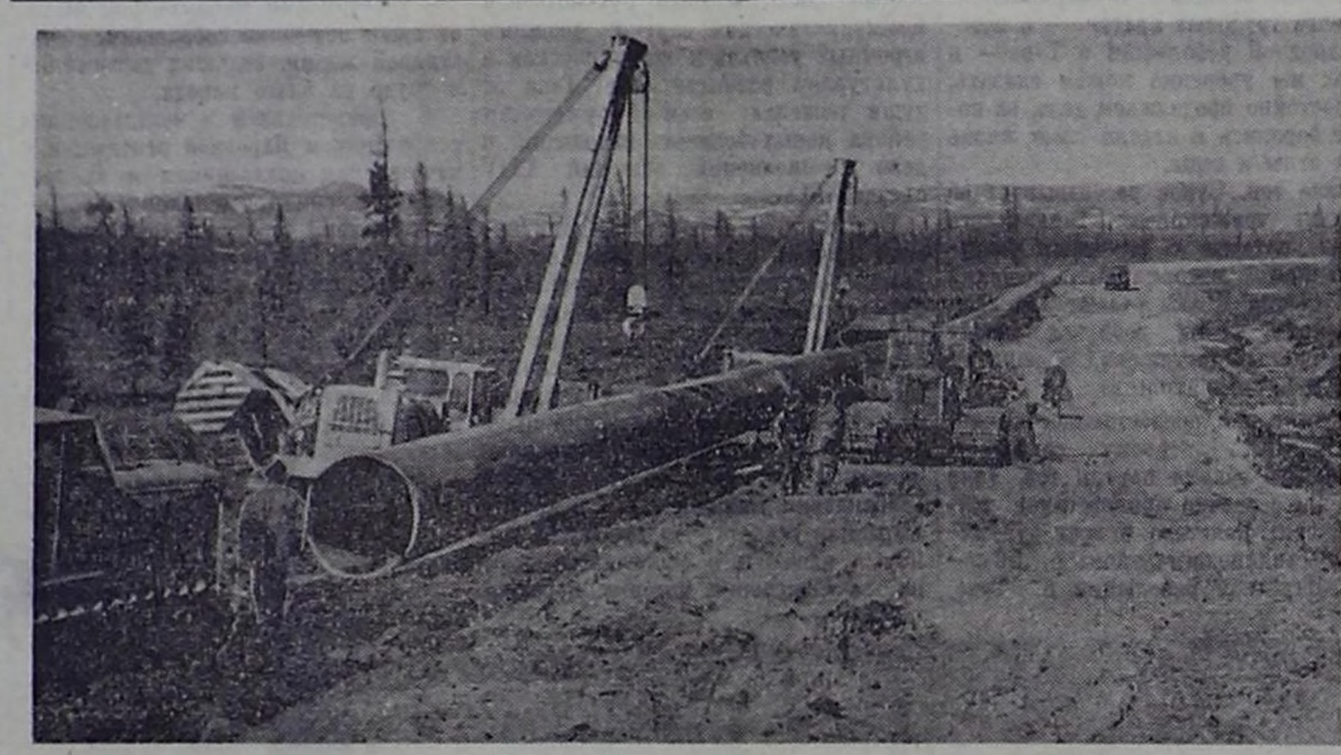
Тюменская область. Сварены вилку первые 35 километров мощного газопровода Надым—Ухта. Диаметр трубы этой новой магистрали — 1,420 миллиметра, протяженность — около 1,200 километров. Трубопровод рассчитан на транспортировку газа при давлении 75 атмосфер. Центральным и западным районам страны он будет передавать с богатейших месторождений Ямало-Ненецкого национального округа десятки миллиардов кубометров природного газа в год. Этот фоторепортаж сделан в горах Полярного Урала на участке трассы, где работы ведет экспериментальное специализированное управление № 5 треста Союзгазспецстрой.
