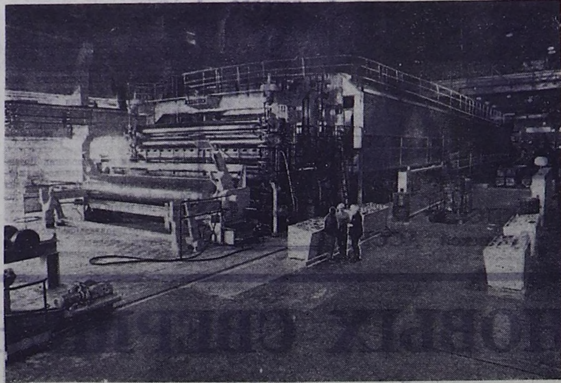
Пермская область. На Соликамском целлюлозно-бумажном комбинате завершён монтаж 12-й быстходной бумагоделательной машины производительностью 114 тысяч тонн газетной бумаги в год. Сейчас идёт регулировка и наладка всех узлов машины. С пуском её в эксплуатацию комбинат станет самым крупным в стране. Он будет вырабатывать 40 процентов всей газетной бумаги. На снимке: общий вид новой быстходной бумагоделательной машины № 12. Фото Е. Загуляева. (Фотохроника ТАСС).
