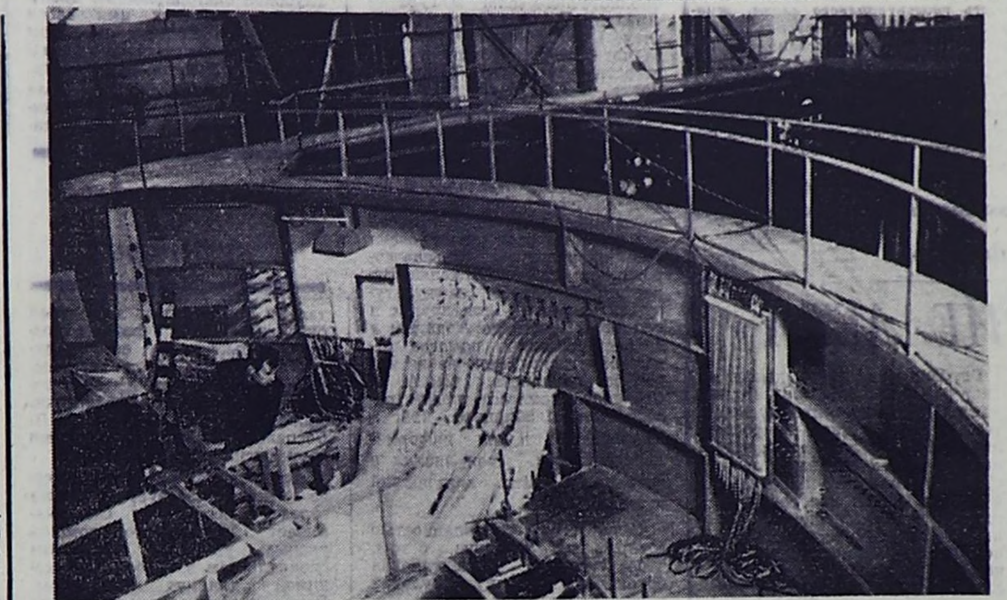
Ленинград. В лаборатории гидравлики, гидроузлов и сооружений научно-исследовательского института гидротехники имени Б. Е. Веденеева проводятся исследования различных вариантов паводковых водосбросов Саяно-Шушенской ГЭС. Ученые, инженеры и техники лаборатории провели сотни экспериментов, цель которых — обеспечить безопасность пропуска паводковых вод реки как во время эксплуатации ГЭС, так и во время ее строительства. На снимке: модель плотин Саяно-Шушенской ГЭС, проводится один из опытов. Фото И. Баранова. (Фотохроника ТАСС).
