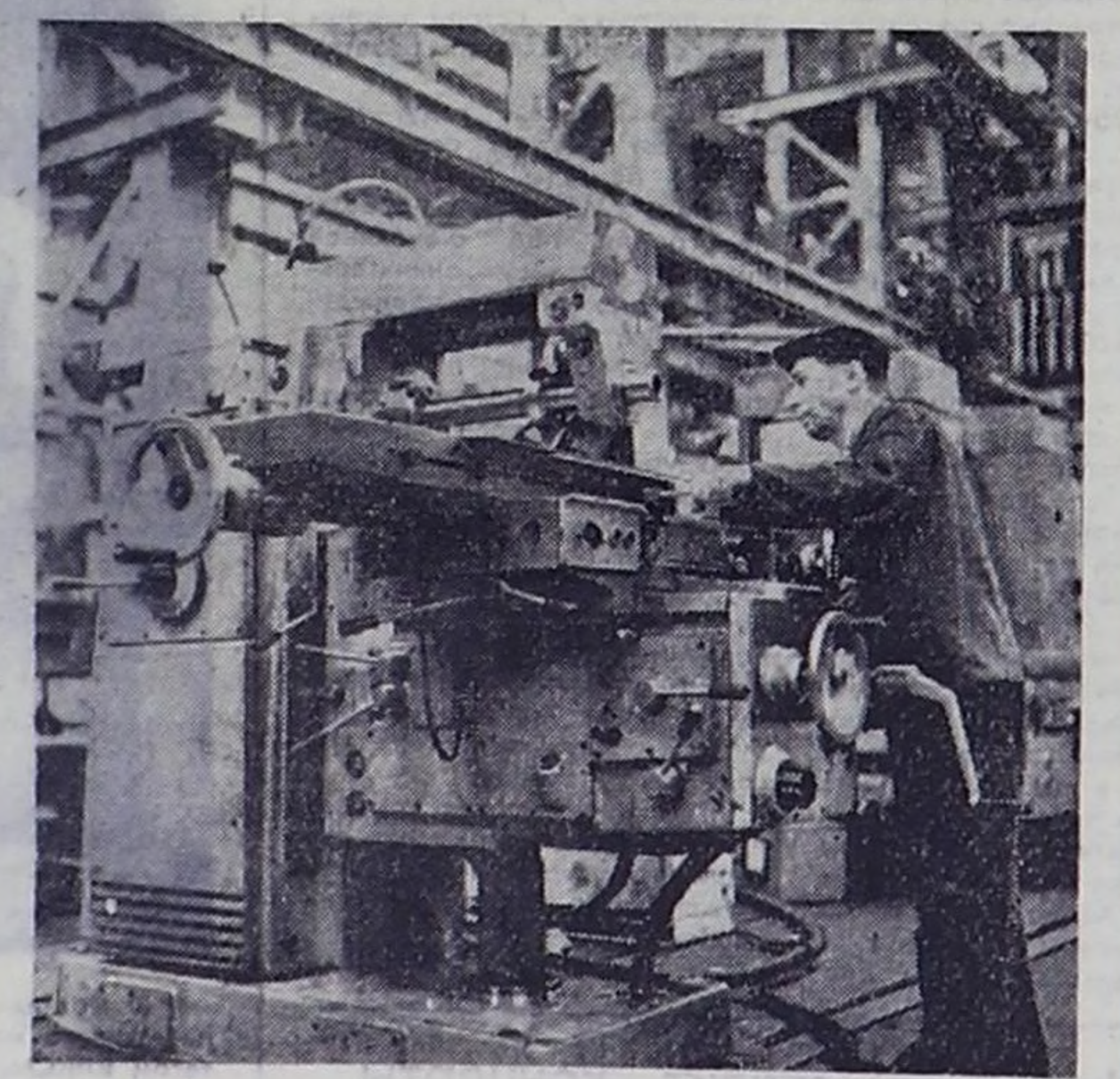
Горький. На станкостроительном заводе изготовлен опытный образец горизонтального консольно-фрезерного станка с системой автоматической регулировки подачи. Точность фрезерования на новом станке в 2 раза выше, чем на других подобного типа, а производительность больше на 30—40 процентов.
