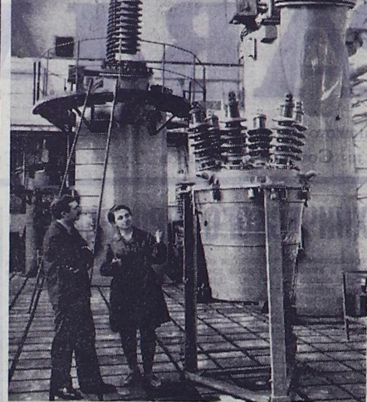
Свердловск. В научно-исследовательском электротехническом институте завода «Уралэлектротрактор» имени В. И. Ленина заканчиваются испытания масляного выключателя на 220 киловольт. Такие выключатели найдут широкое применение при строительстве высоковольтных линий электропередач. На снимке: конструктор А. Ф. Буйлов и инженер-исследователь Э. А. Барвинова в лабораториях механических испытаний масляных выключателей на 220 киловольт. Фото А. Грахова. (Фотохроника ТАСС).
