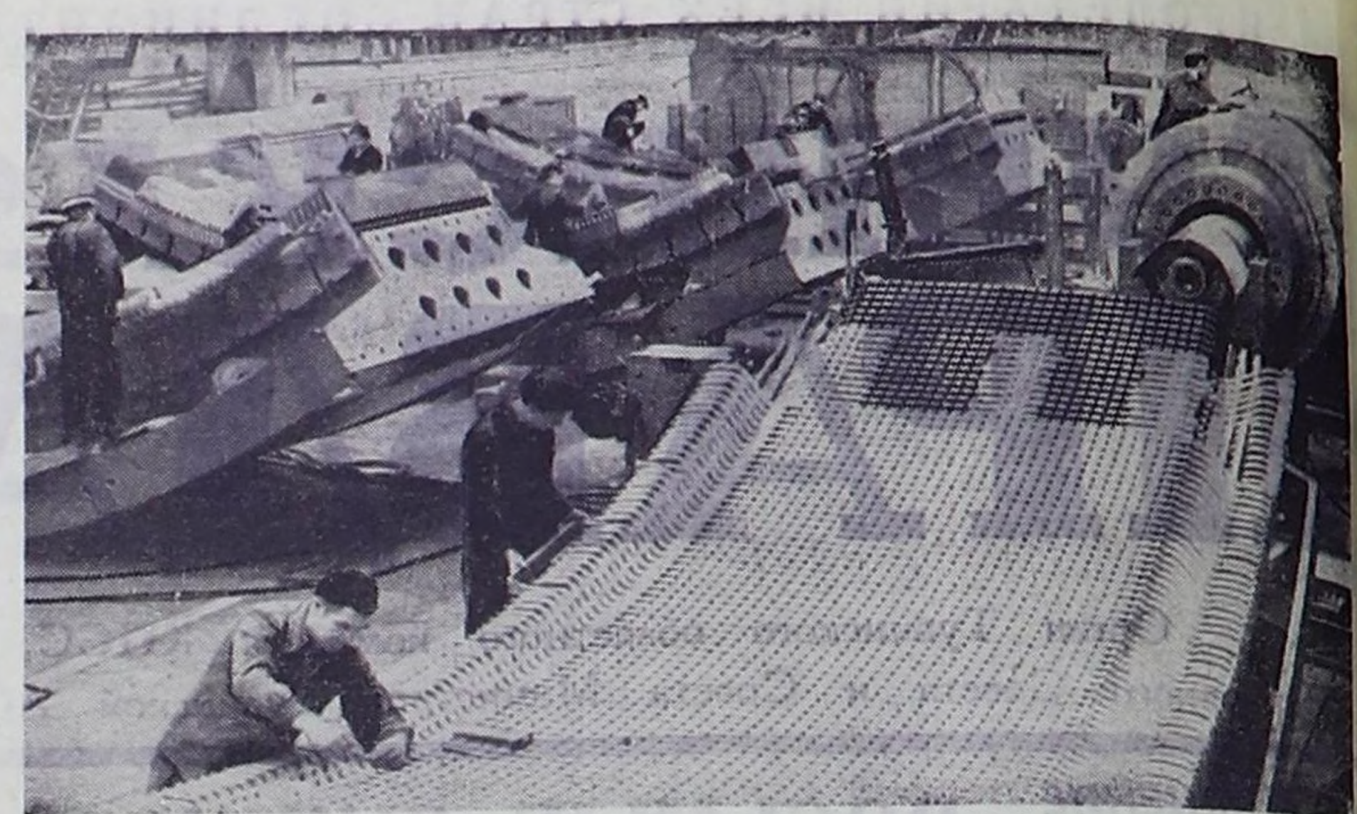
Ленинград. Машиностроители объединения «Электросила» изготавливают мощные гидрогенераторы для Дунайской ГЭС «Железные ворота», строящейся совместно румынскими и югославскими специалистами.
