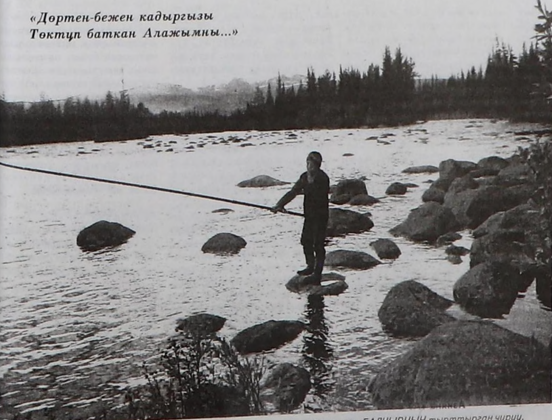
«Имиртинде балыктаашкын».
