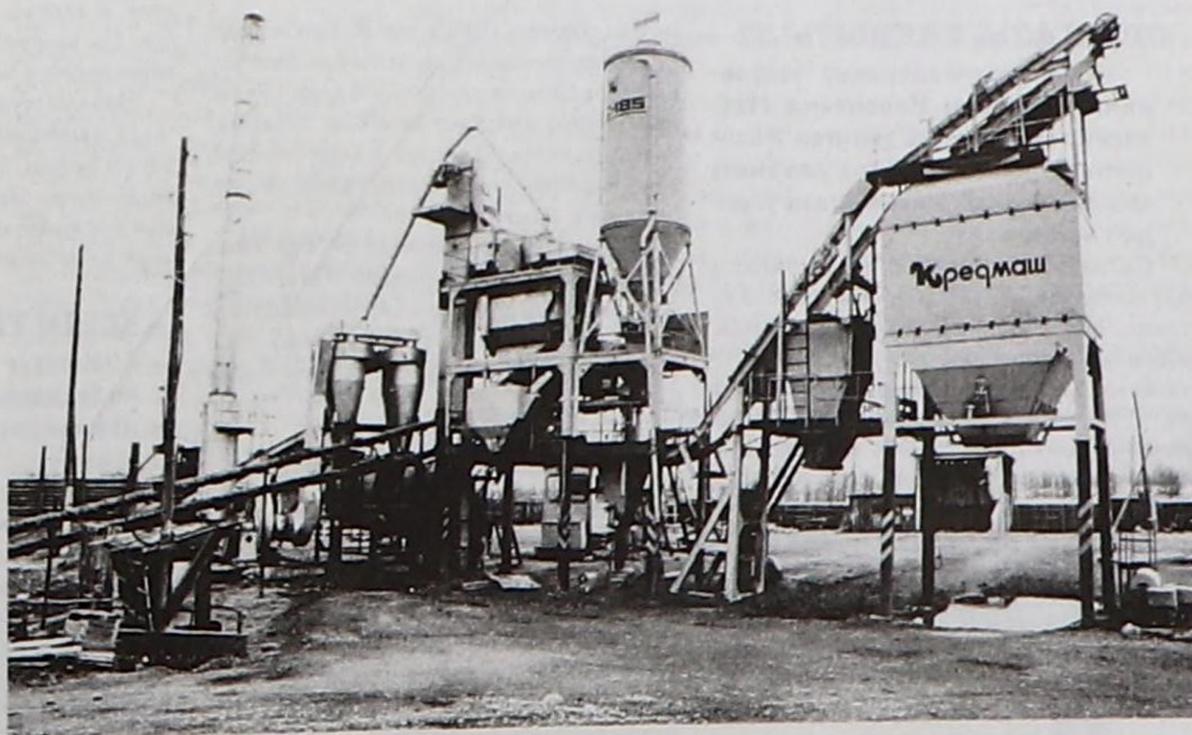
Асфальт бүдүрер завод.
