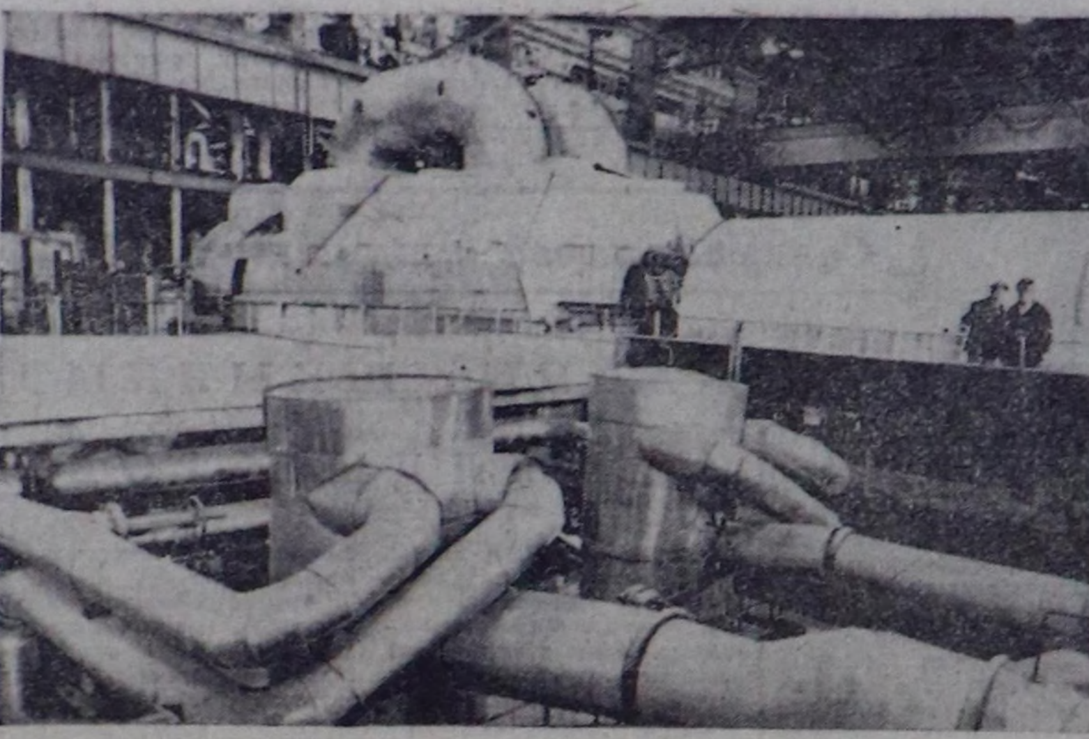
ЧУРУНГА: Барын Сибирьде нефть га-зы-биле ажаллаар Сургут ГРЭС-тин маши-на залы. Бо станция беш чылдын бирги чылдан өгөлэп 45 млрд. кет-шак элек-троэнергияны ажаллап кылган. СЭТА-ның фотоу.
