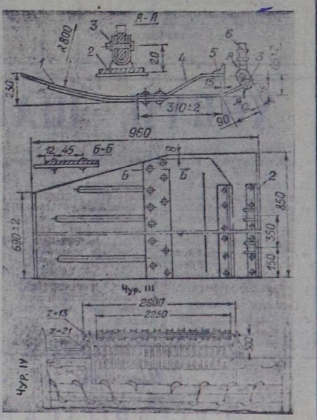
Чурук I. В. Морозовтун чогааткан аргазы. 1—граблинниң трубазы; 2—кол граблинниң салаалары; 3—немелде граблинниң салаалары; 4—шпидин. Чурук II. Салаа чок кезер аппарат. Чурук III. Тавычаларны кожа кылдыр кестирер-биле ЖВН-6 жаткага немей кылган тургузуу. 1—шит; 2—полоса; 3—скоба; 4—козырек; 5—уголок; 6—тускай эриал. Чурук IV. Немелде салаа барабанын бөдүрүчүлүүн схемасы.
