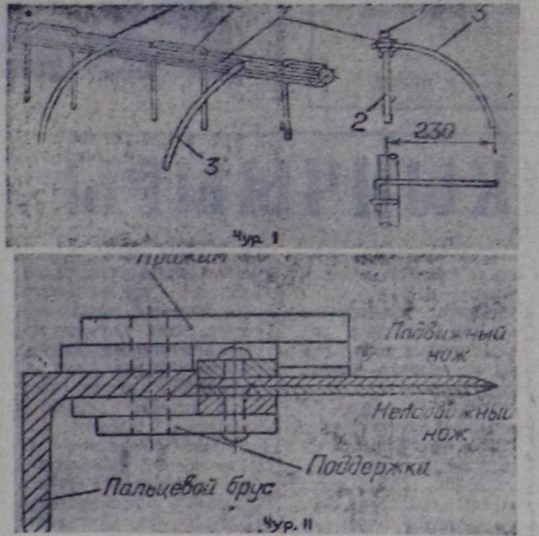
Чурук I. В. Морозовтун чогааткан аргазы. 1—граблинниң трубазы; 2—кол граблинниң салаалары; 3—немелде граблинниң салаалары; 4—шпидин. Чурук II. Салаа чок кезер аппарат. Чурук III. Тавычаларны кожа кылдыр кестирер-биле ЖВН-6 жаткага немей кылган тургузуу. 1—шит; 2—полоса; 3—скоба; 4—козырек; 5—уголок; 6—тускай эриал. Чурук IV. Немелде салаа барабанын бөдүрүчүлүүн схемасы.
