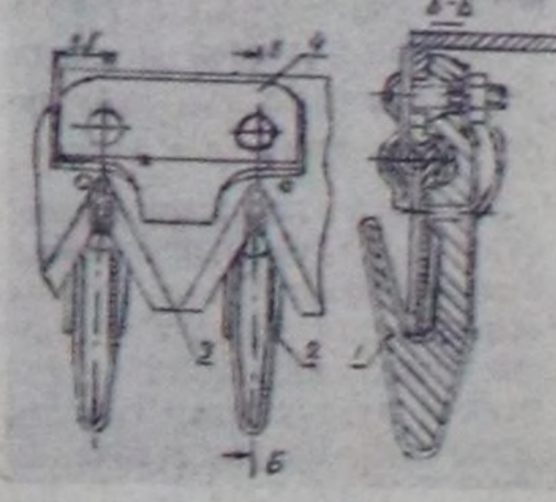
«ЖВН-6» жатканын бозба-зырапгажыттыган болжам-жы. 1—дини; 2—дуур кезер пластина; 3—бис; 4—чы-пыр базар баскыш.
