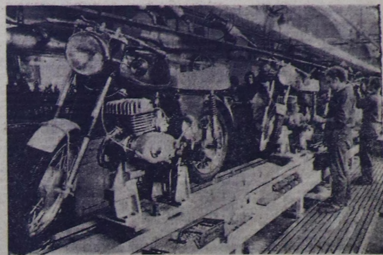
ГДР-ниң Цшопауда заводу 250 кубитиг сантиметр класстың орук мото-цилинниң хөй хөвирин дыка чазартып алган. Чаа хөвирин ол мотоцилин «ТС-250» деп адаар. ЧУРУНТА: «ТС-250» эптээр конвейерде. АДН — СЭТА-ның фотозу.
