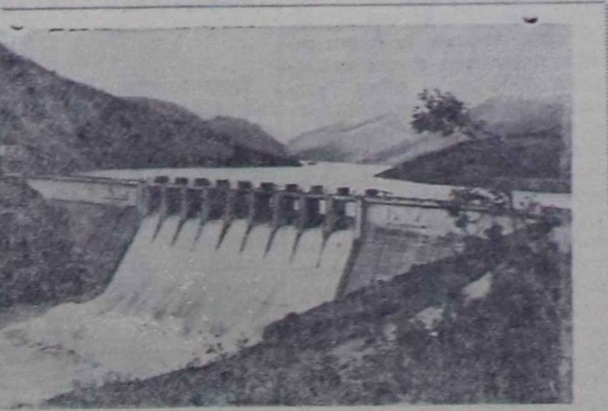
Болгарияның Улус Республикасы. Чуртун муруу чарымында Чен Родопылар дагырында Болгарияда гидротехниктиг туз-ларын өн улустарынын бирөөн—«Студен кладевец» туу-дооскан. Ол гидробадынын тузугулары даг хем Арданың уу-ну узуну 338 метр болгаш бедни 72,5 метр платина-биле боопкан болгаш узуну 29 километр суг шыгжаарын тургускан. Маа 60.000 киловатт күчүлүг гидроэлектростанцияны база туткан. Чурунта: «Студен кладевец» деп суг шыгжаары. СЭТА-ниң фотохрониказы.
