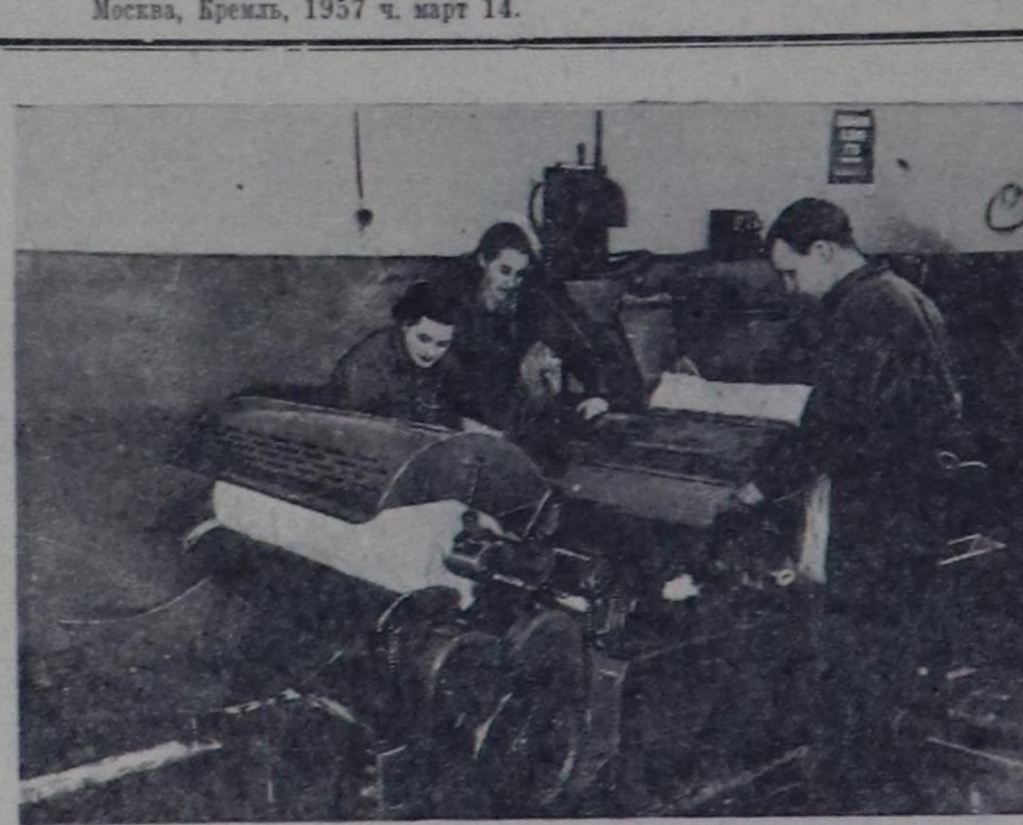
Ленинград. Хөвөң кылларында хөвөңг «МВЧ»-100 деп хөвөң дырап кыллар чаа машинаны «Вулган» заводтун бөлүк конструкторлары чогадып кылган. Ол машина шақта 40 килограмм чедир хөвөңни дырап бүдүрүчүлүгү, машина чаа техника-биле хандырылган. Чурунта (солгай талазында оң талазында): слесарь-механик М. Е. Семенов, инженер-конструкторлар Г. С. Сахаров болгаш А. З. Шерман оларның чаа машинаны шыгалада белеккен турары. Фото А. Михайловтуу. СЭТА-ның фотохроникасы.
