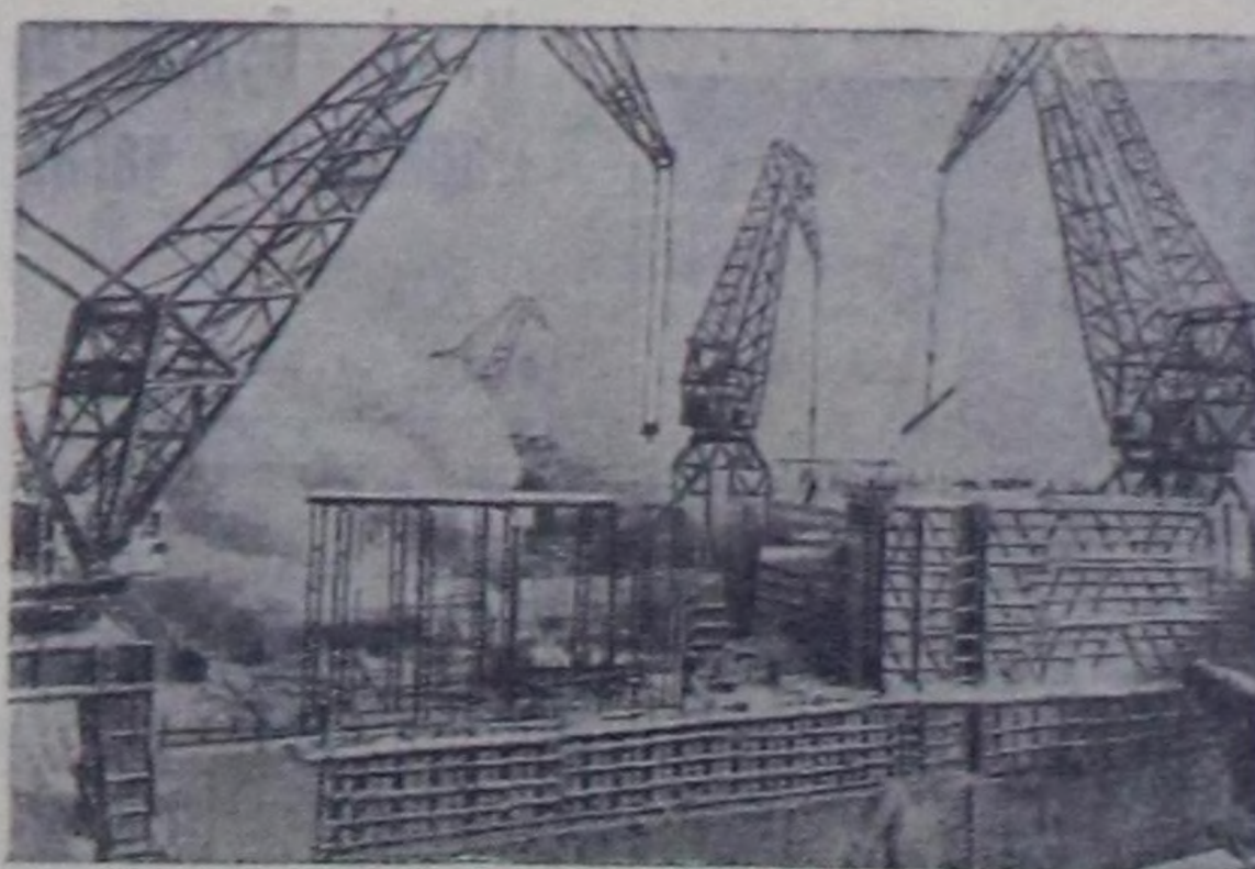
Иркутск. Иркутск ГЭС-тин бажыны улам-на бедип турар. Чымылаа сова турээ-даа, туудуужулар бетон салырып урдузуп турар. Блоктары бус болгаш алектри-биле чымылаа, бетон массазын чымылаа байдал-биле берип турар.
