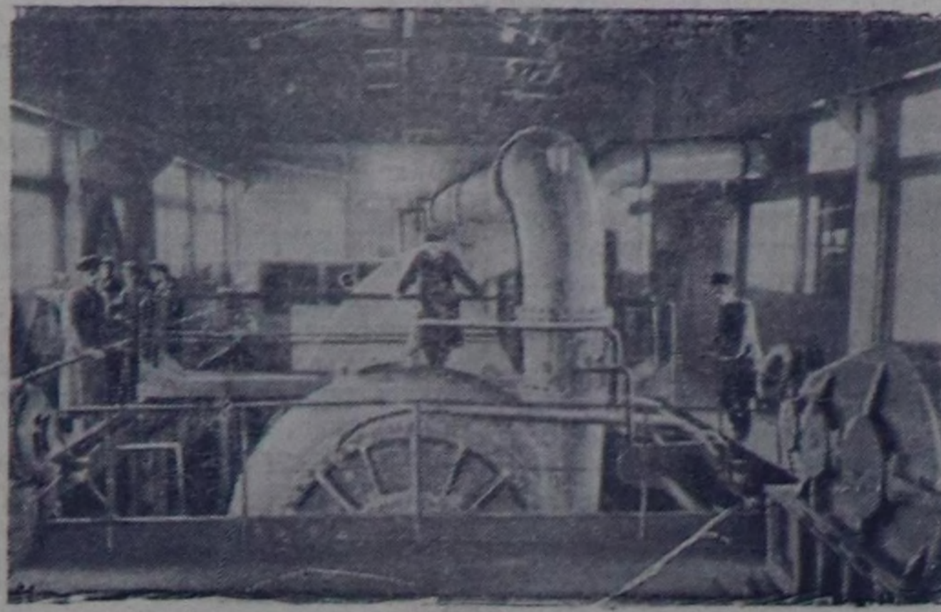
КУЙБИШЕВГИДРОСТРОЙ.—Делегейде эн-не улуг хемчээлдиг доврак сордурар «Сталинградский-1» деп терини күштүг машина улуг тудугда чеде берген. Ол 4 километр хире узун дурттуг черге бир шактын дургузунда мун-мун кубометр довракты казып шыдаар.
