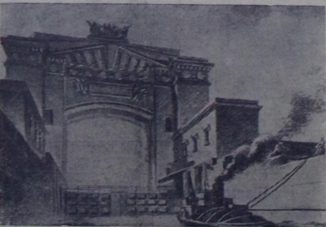
Цимлянсканын суг бедиринде шлюзтуң кирер экинин архитектурлуг төлөвилеги. „Советский Союз“ деп журналдан.
