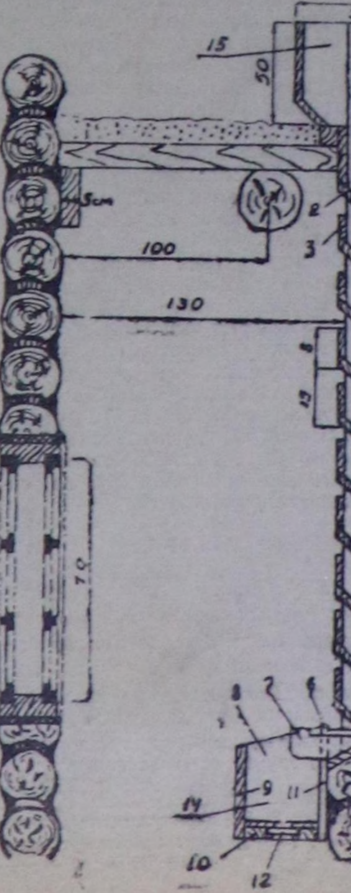
Чурук № 3. Кургадылга секциясы. 1. Секциянын тетивазы. 2. Ийленчек полочка. 3. Дорт полочка. 4. Төгөр полочка. 5. Козырек. 6. Секциянын задвижкасы. 7. Углар задвижка. 8. Кобылка. 9. Хааржактын муриуку ханазы. 10. Хааржактын дуву. 11. Хааржактын артыкы ханазы. 12. Хааржактын задвижкасы. 13. Секция адаанда ыш. 14. Кургаткан тараа урар хааржак. 15. Шык тараа урар бункер.
