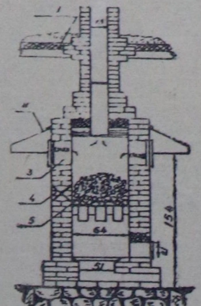
Чурук № 2. Каменка деп печка (чара кескини). 1. Потолок, 2. Козырек, 3. Изиг агаар үнер дыдык чер, 4. Печканын даштарын аштаар чер, 5. Даштары.
